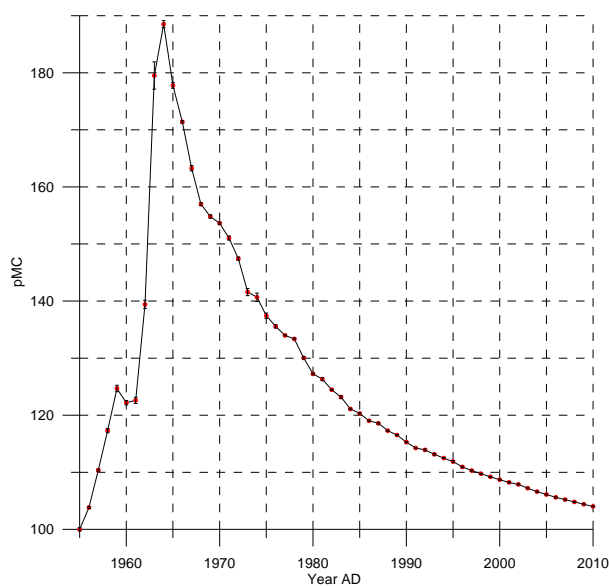
Rys. 3. Zawartość węgla ^{14}\text{C} w powietrzu atmosferycznym w latach 1955-2010
